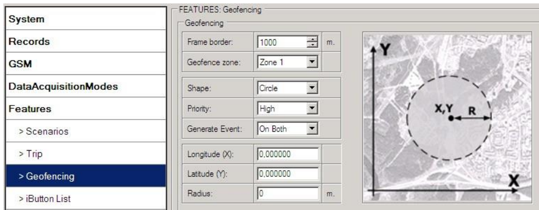
Рис. 32. Конфигурирование геозоны.
